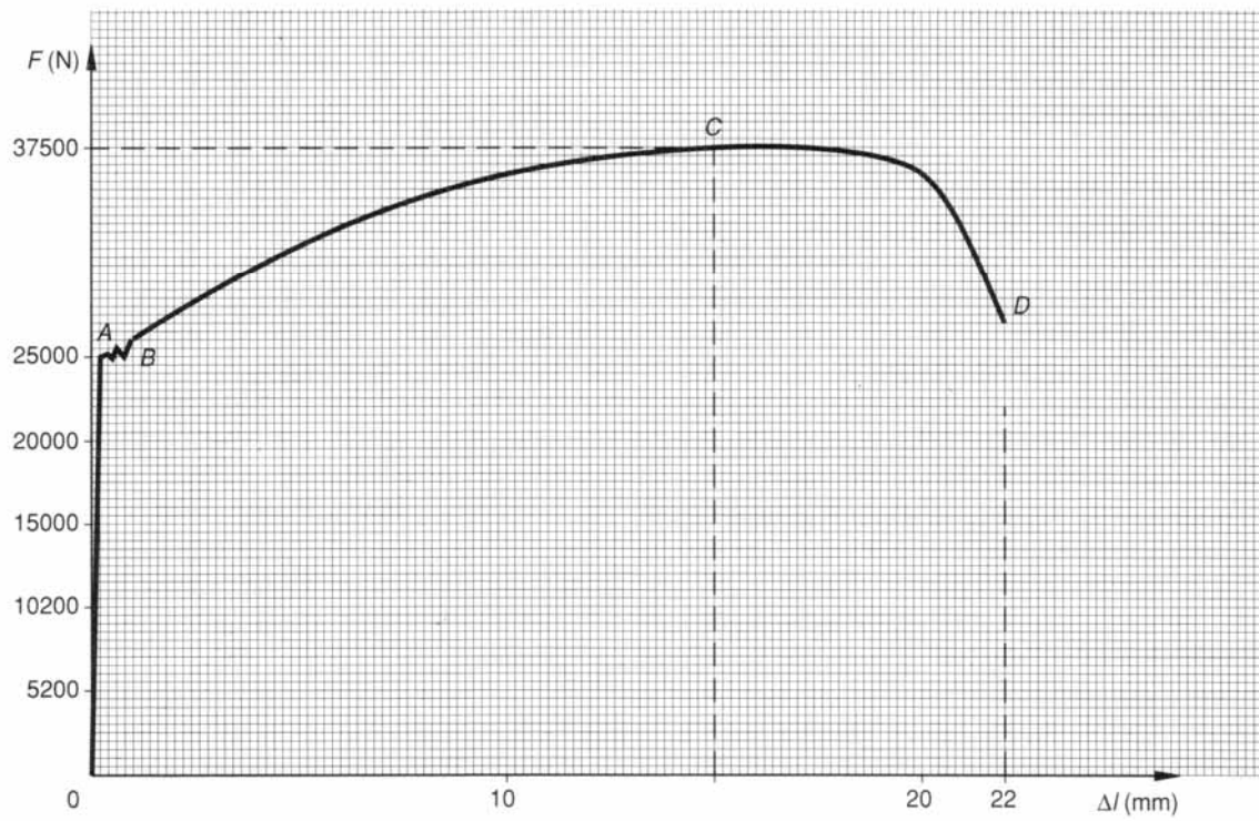
Enregistrement d'un essai d'extension (acier E30).
